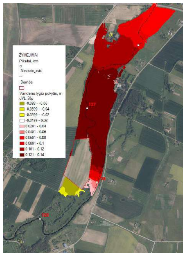
3.3 pav. 50% tikimybės potvynio maksimalių vandens lygių pokyčiai dėl apsauginių dambų poveikio
