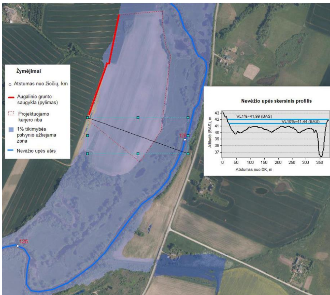
11 pav. Projektuojamo pylimo padėtis po atliktos detalios analizės ir Nevėžio upės skersinis profilis
