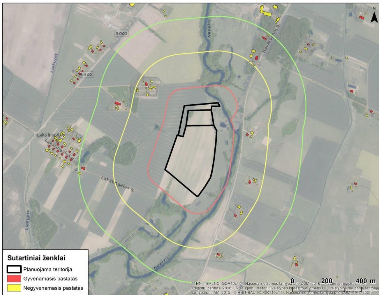
45 pav. Artimiausių gyvenamųjų ir negyvenamųjų pastatų situacijos schema
