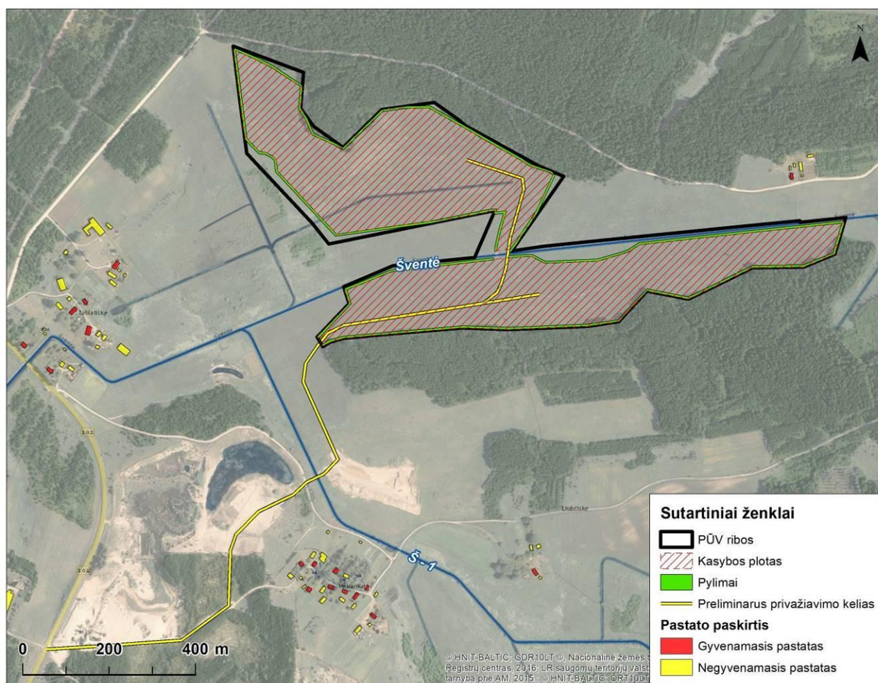
47 pav. Planuojama situacijos schema
