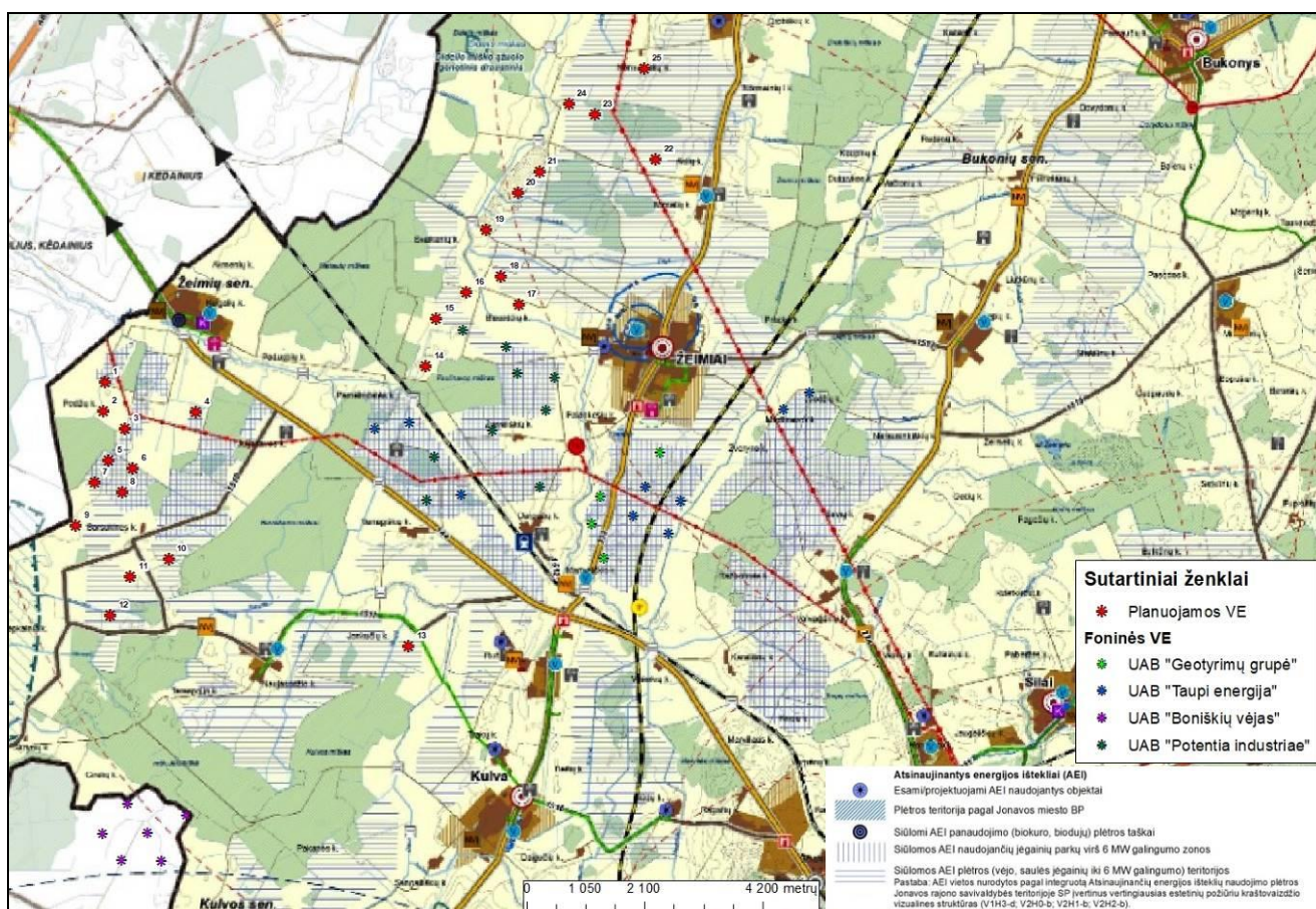
4 pav. Ištrauka iš Jonavos rajono savivaldybės teritorijos bendrojo plano susisiekimo ir inžinerinės infrastruktūros brėžinio
