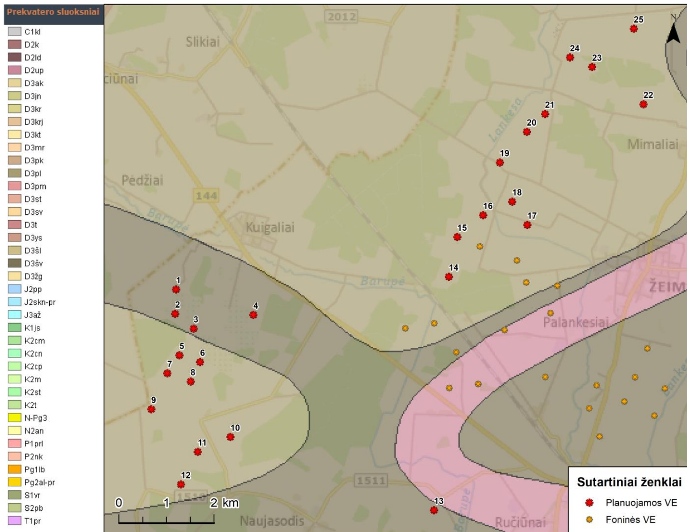
17 pav. Prekvarterio geologinio žemėlapio ištrauka 11
