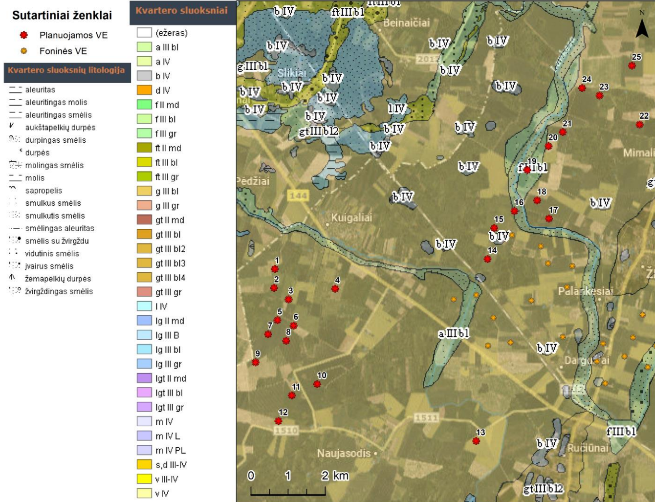
18 pav. Kvartero geologinio žemėlapis ištrauka 12
