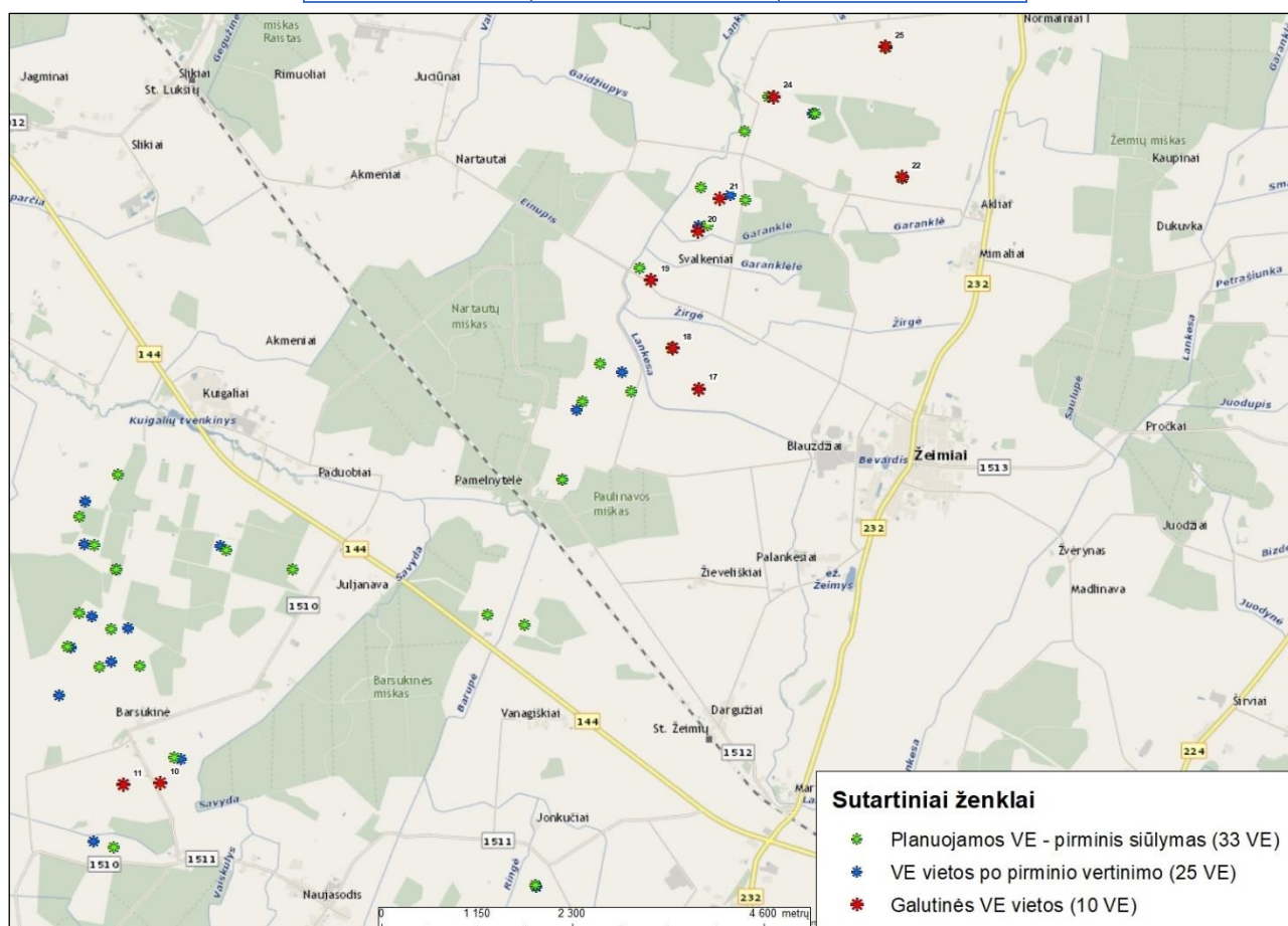
2 pav. Planuojamų VE vietų ir skaičiaus pokyčio vizualizacija (atsisakyta VE11)
