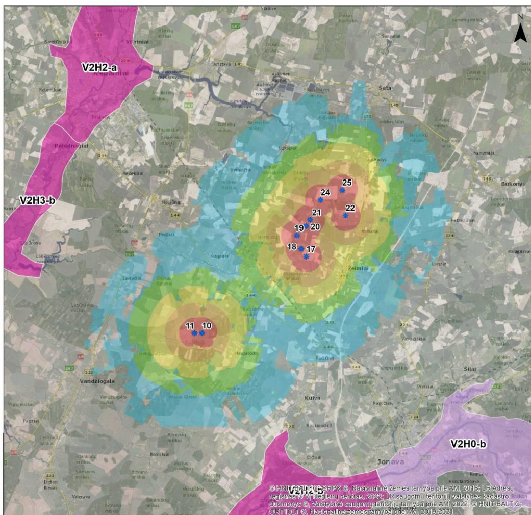
28 pav. Ypač saugotino vizualinio ir estetiško potencialo arealai ir vietovės VE kraštovaizdžio vizualinio poveikio zonų atžvilgiu (atsisakyta VE11) (vertinant pagal vertikalų matymo kampą)
