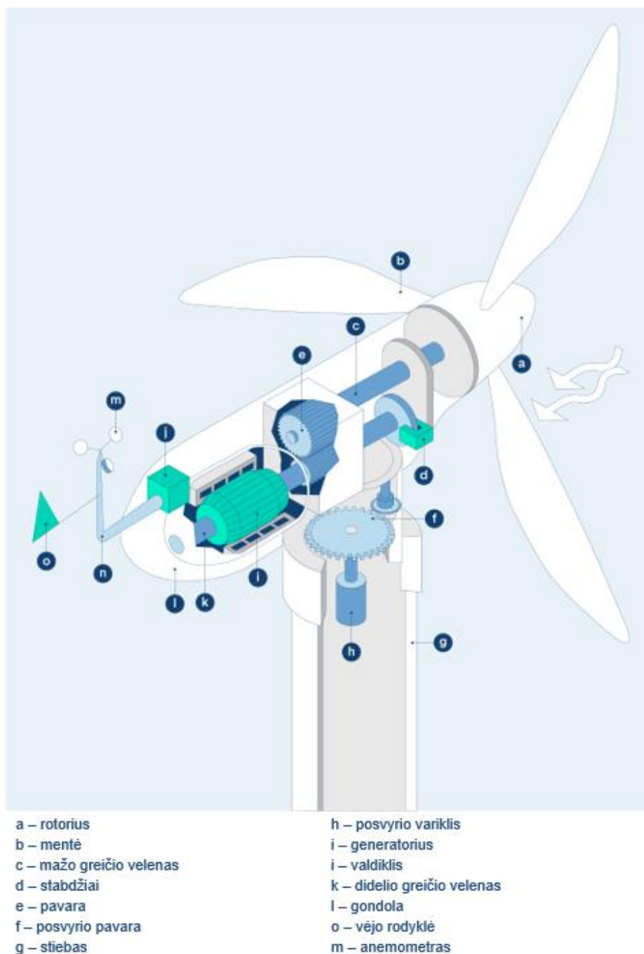
2 pav. Vėjo elektrinės konstrukcija ir veikimo principas (atsisakyta VE11)
