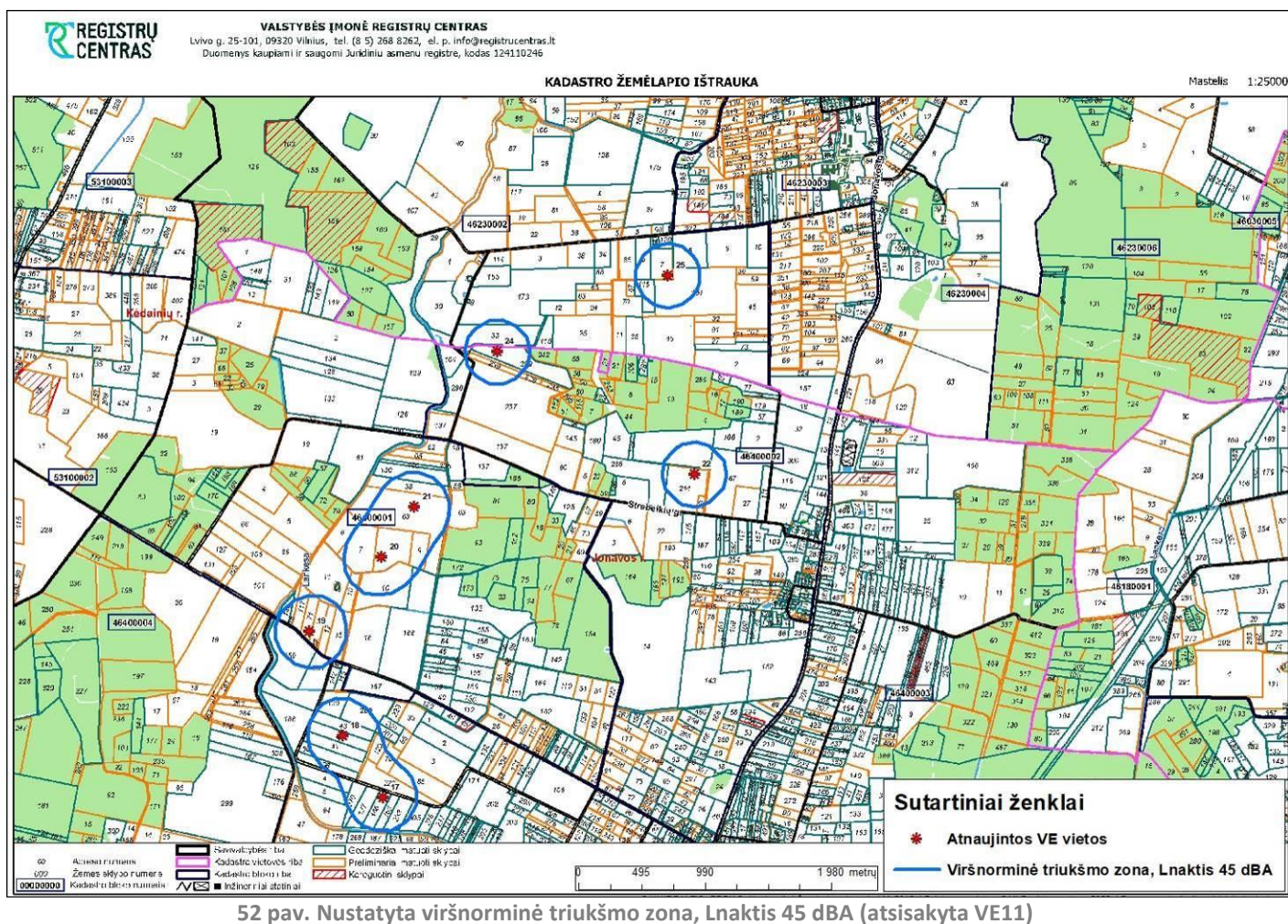
52 pav. Nustatyta viršnorminė triukšmo zona, Lnaktis 45 dBA (atsisakyta VE11)
