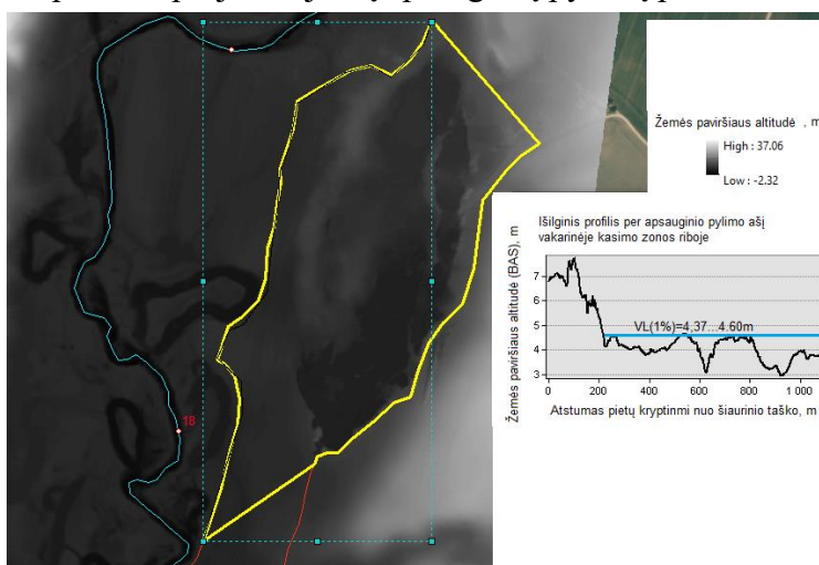
2 pav. Žemės paviršiaus aukščiai ir potvynių vandens lygiai vakarinėje kasimo zonos riboje
