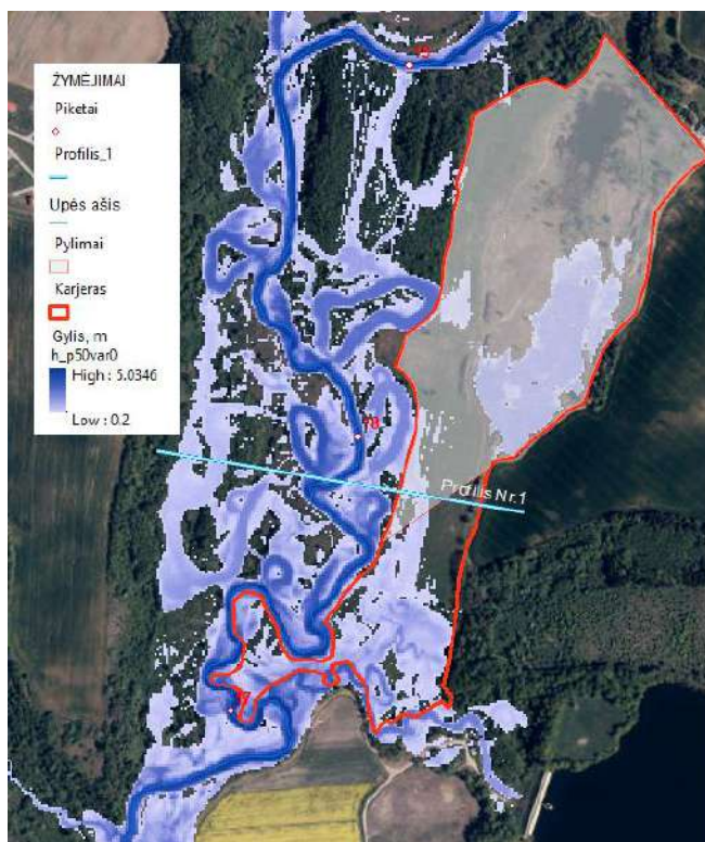
3.2 pav. 50% tikimybės potvynio gyliai ir apsejami plotai „0“ batimetrijos variante
