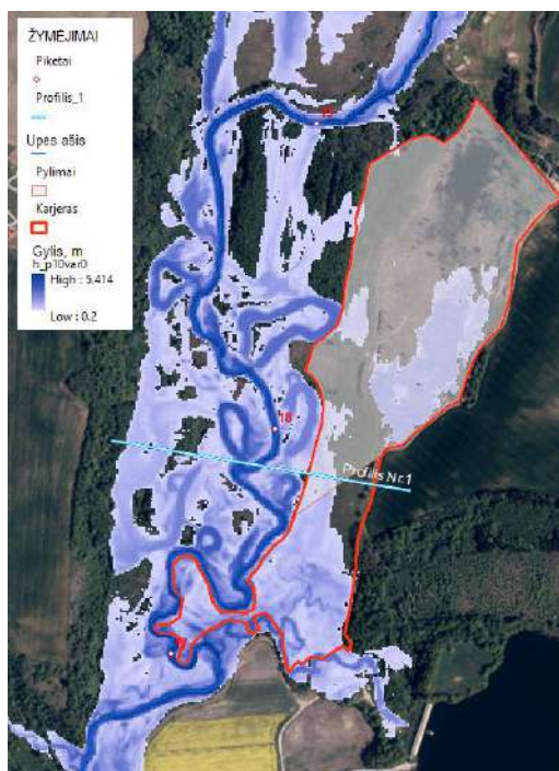
3.3 pav. 10% tikimybės potvynio gyliai ir apsejami plotai „0“ batimetrijos variante
