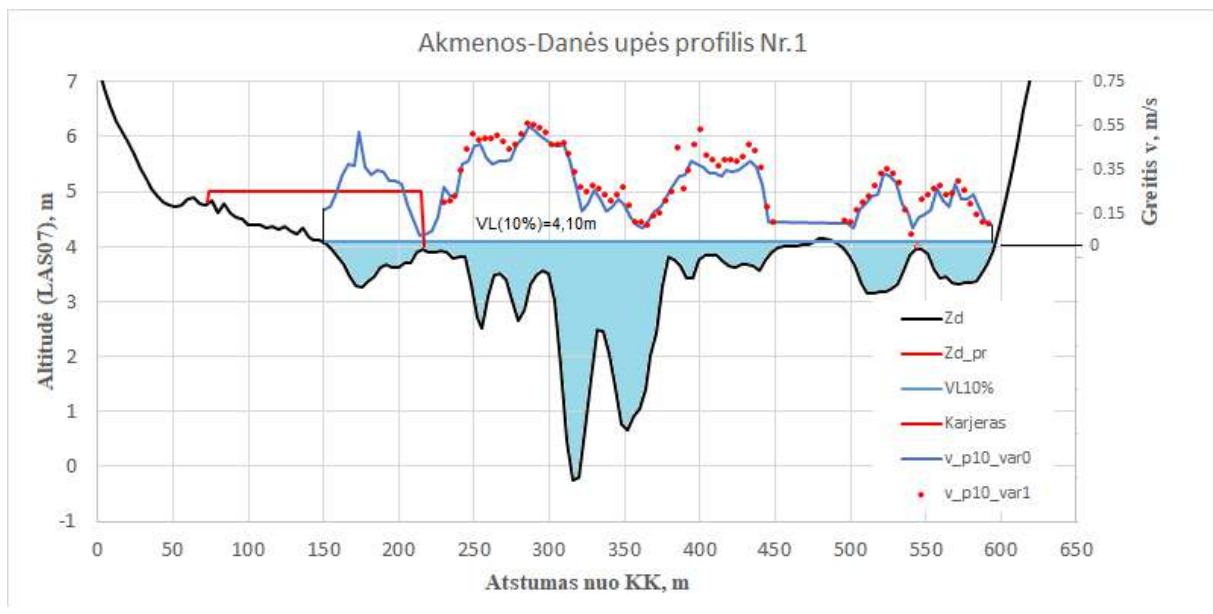
3.14 pav. 10% tikimybės potvynio tėkmės greičiai upės profilyje Nr.1.
