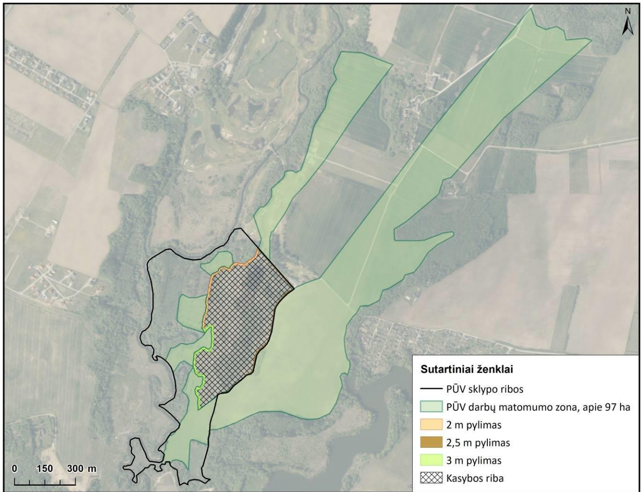
16 pav. Nustatyta preliminarai PŪV darbų matomumo zona, įvertinant augmeniją, pastatus ir reljefą
