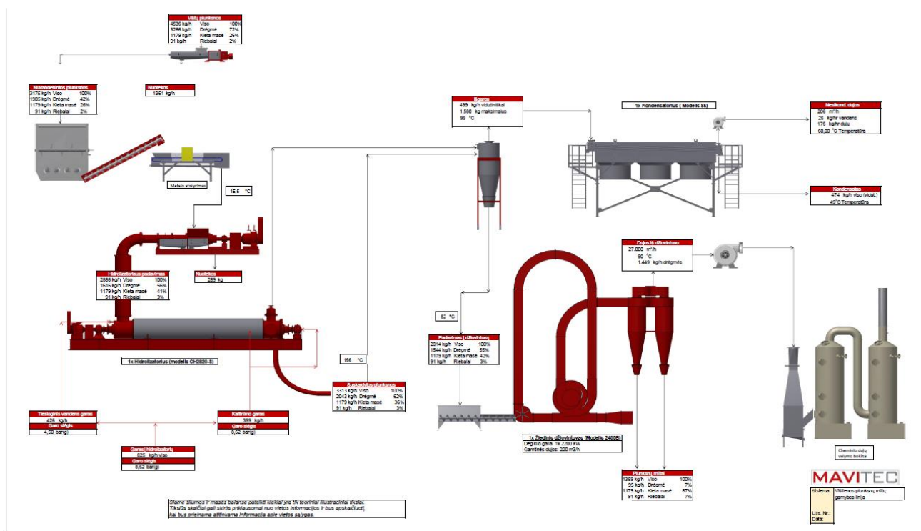
2 pav. Plunksnų apdorojimo technologija
