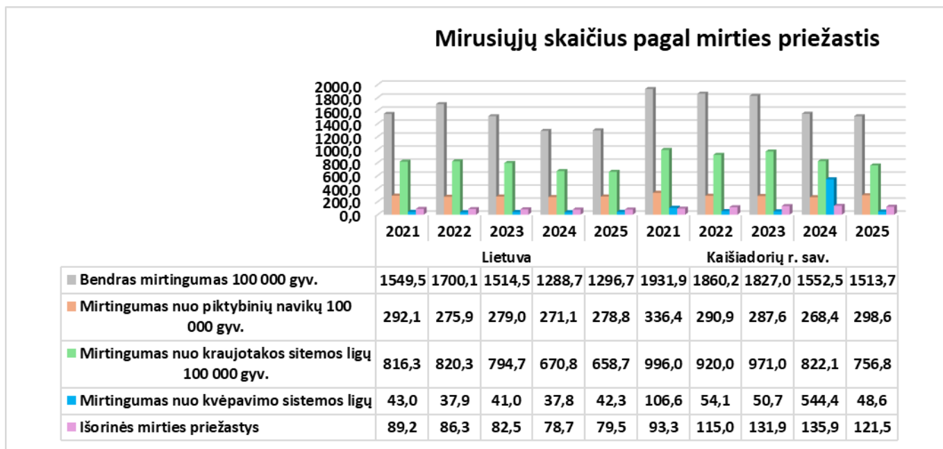
19 pav. Mirties priežasčių pokytis Kaišiadorių r. sav. bei Lietuvoje tenkantis 100 000 gyventojų
