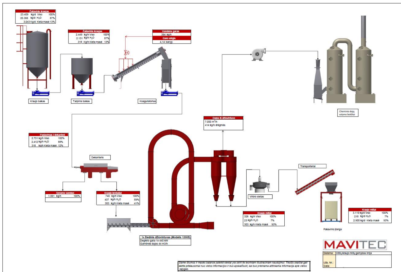
3 pav. Kraujo apdorojimo technologija
